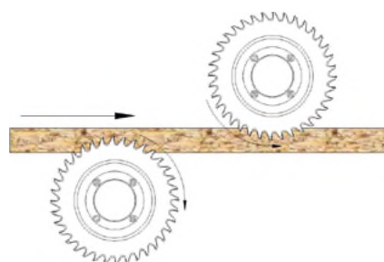
Feed speed for double hogger Vitesse d'avance pour déchiqueteur double
