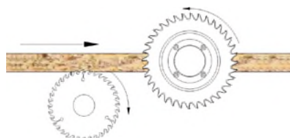
Feed speed for scoring /hogger Vitesse d'avance pour Inciseur/déchiqueteur
